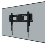
WL30-750BL16 Beeldformaat: 42-86" Capaciteit: 125 kg VESA: 100x100 - 600x400
