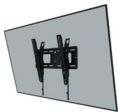
WL35-750BL14 Beeldformaat: 32-75" Kantelen: +15°/-15° Capaciteit: 100 kg VESA: 100x100 - 400x400
