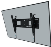
WL35-750BL16 Beeldformaat: 42-86" Kantelen: +15°/-15° Capaciteit: 125 kg VESA: 100x100 - 600x400
